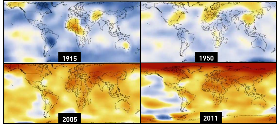
Cartes du réchauffement climatique (source : Nasa) Echelle : les différences de températures en degrés Celsius.
